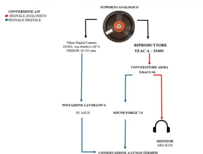
Figura 1 Il processo di riversamento attuato per le bobine
